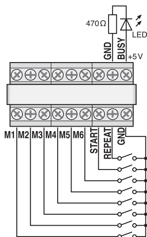
④ branchement pour une gestion à distance
