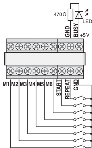
④ conexión para control remoto
