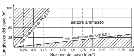
Fig. 5 Sezione del cavo richiesta per il loop ad induzione
