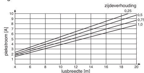
Figuur 7 Piekstroom in de inductielus
