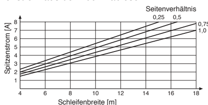
Abb. 7 Spitzenstrom in der Induktionsschleife
