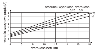
Rys. 7 Wartość szczytowa prądu w pętli indukcyjnej
