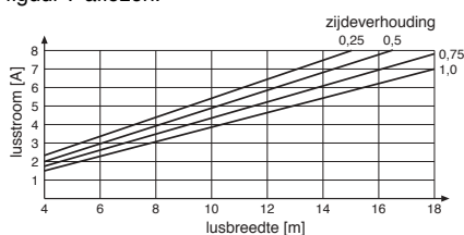
Figuur 7 Piekstroom in de inductielus
