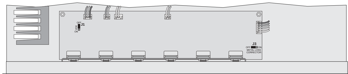
Rys. 8 Przewody potężeniowe J1 i J3
