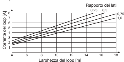
Abb. 7 Corrente di picco nel loop ad induzione
