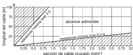
Esquema 5 Sección de cable cruzado requerida para el loop de inducción
