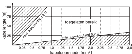
Figuur 5 vereiste kabeldoorsnede voor de inductielus
